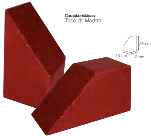
KTT012 TACOS MADERA GDE CAMION 13cm X 13cm x 25cm – X2
