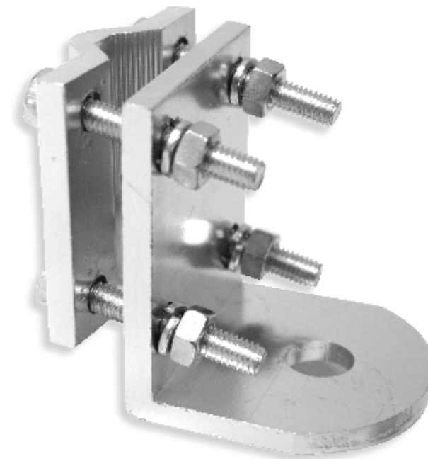
AND060 BASE ANTENA PARA ESPEJO LATERAL 4 TORN VERTICAL X1
